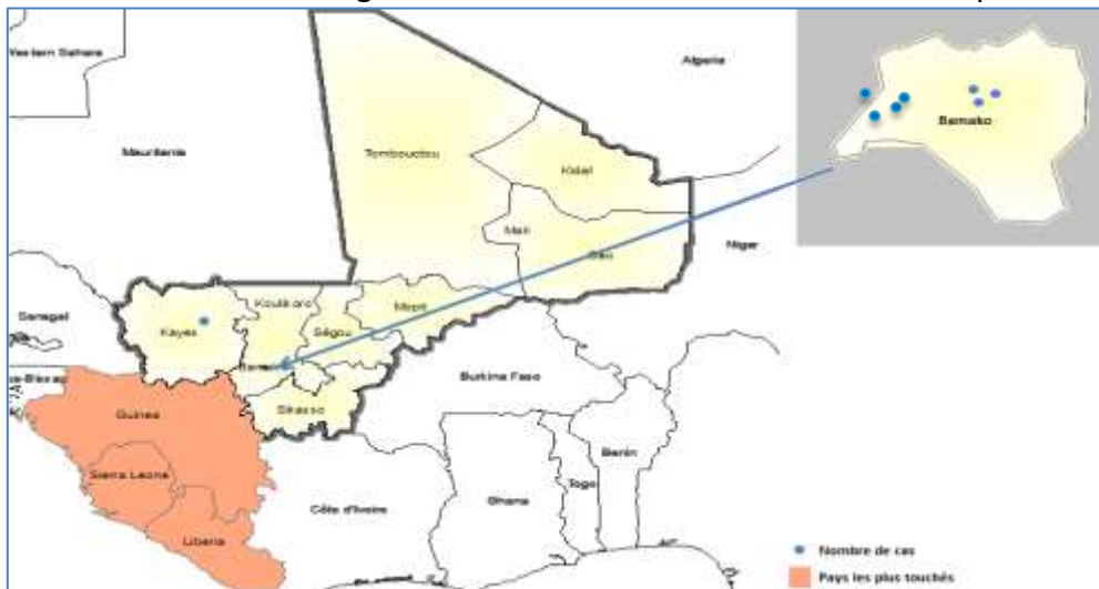
Localisation des cas confirmés (7) et probable (1) de la maladie à virus Ebola au Mali.
